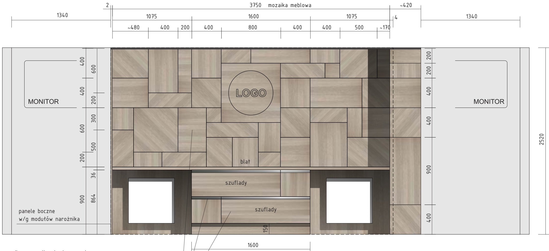
ŚCIANA Z MOZAIKĄ W HOLU GŁÓWNYM 1:25
